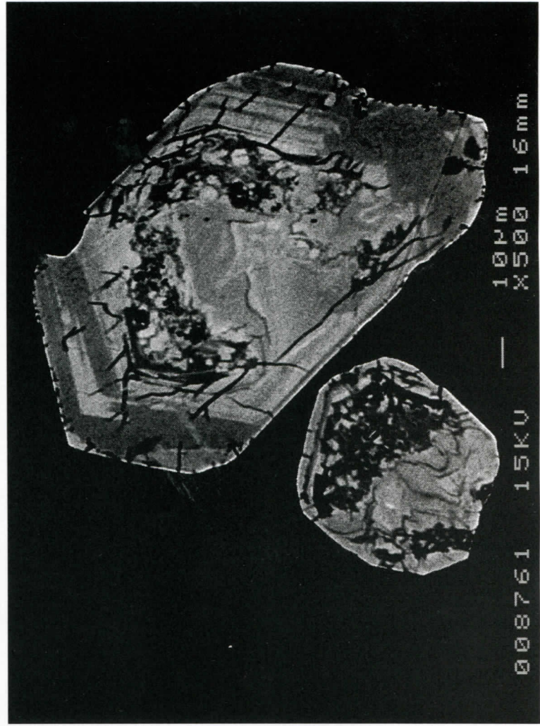
MA5-61a 'Def.' texturatus zircon
