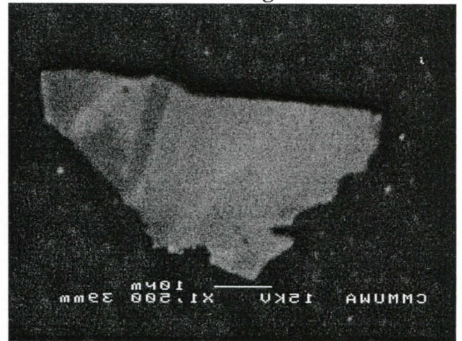
Zircon 9
