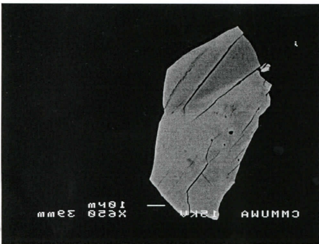
Zircon 11
