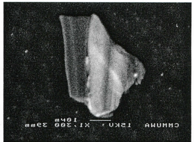
Zircon 10
