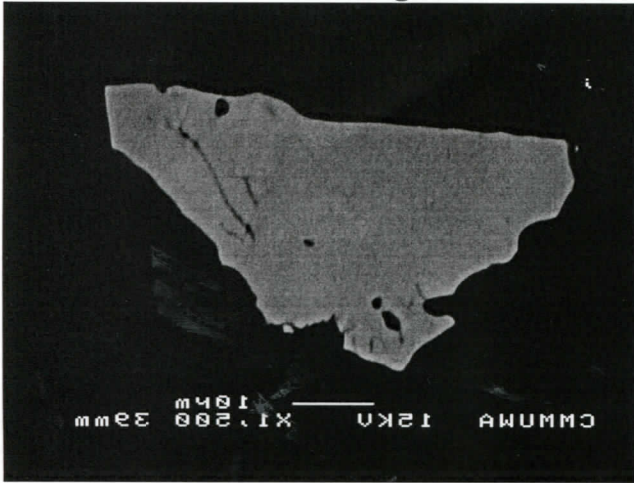
Zircon 9
