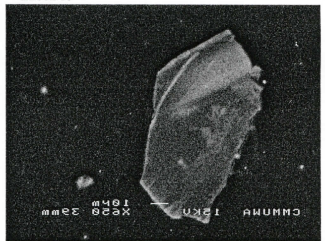
Zircon 11
