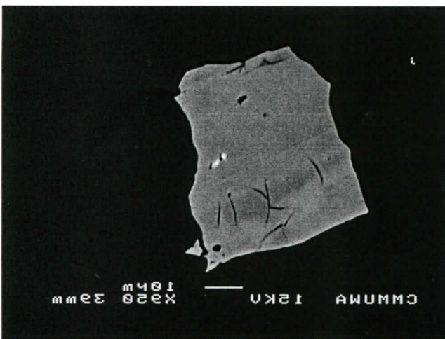
Zircon 12
