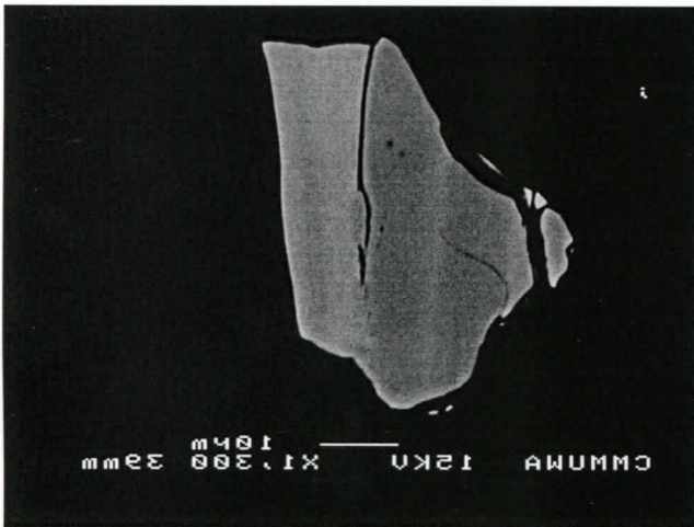
Zircon 10
