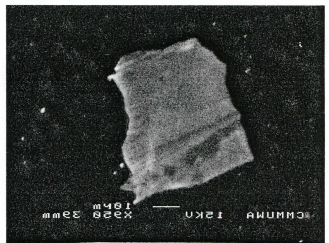
Zircon 12
